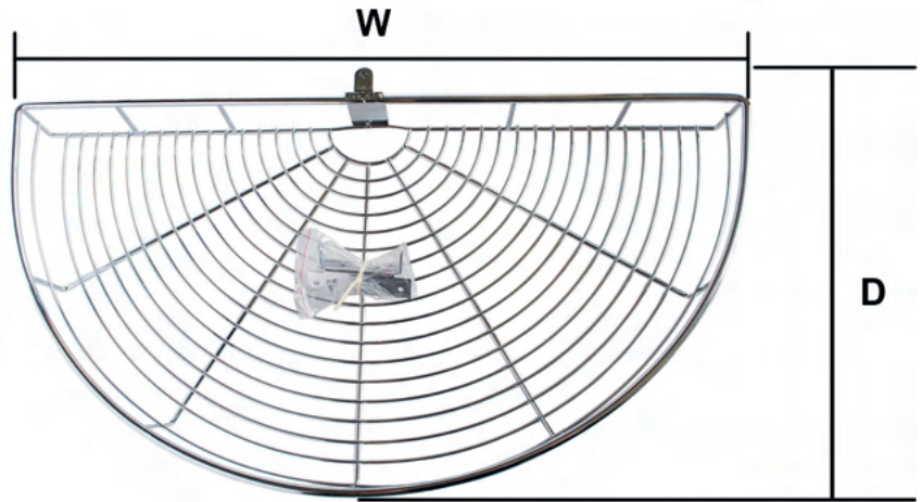
002-SSB-30"
