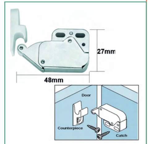
Mini Latch (S) 019-021-001
