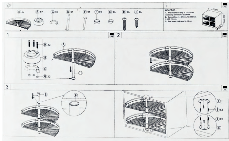
002-008-180
