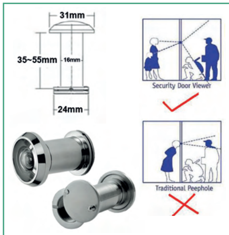
A200 Deg Door Viewer Chrome StG-DV-PB
